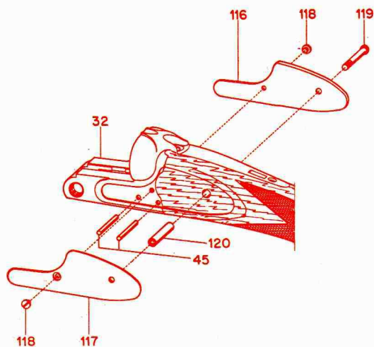
FINTE CARTELLE DUMMY SIDE PLATES CONTRE PLATINES
